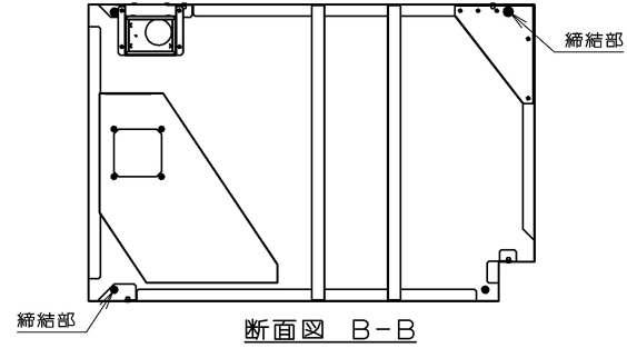
断面図 B-B
