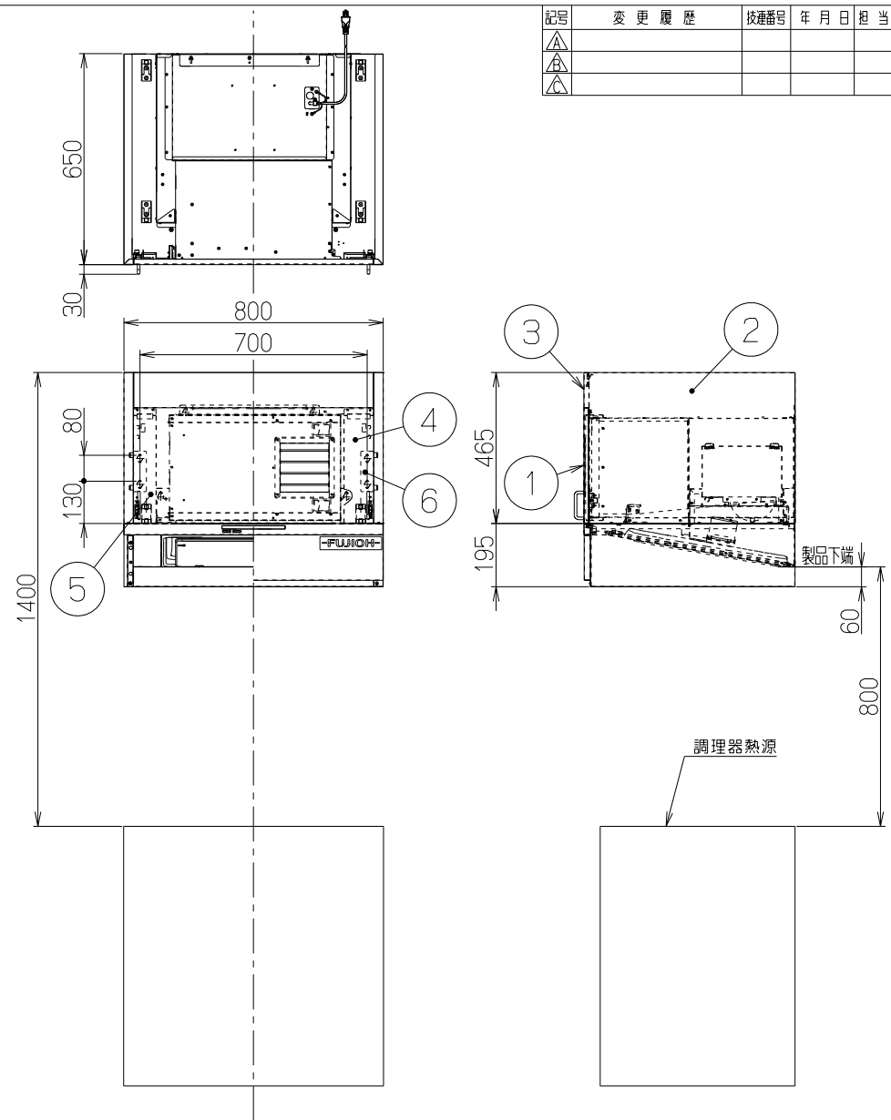
取付図
